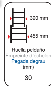
Detalle peldaño Détail marche Detalhe degraus
